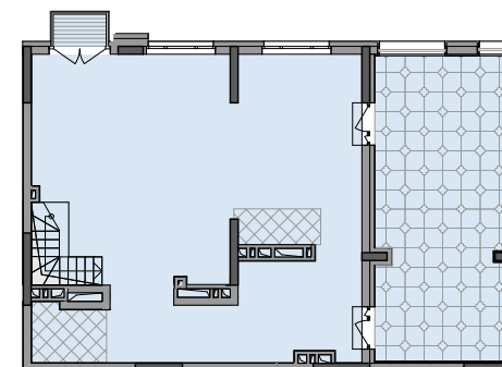
ІІ рівень
