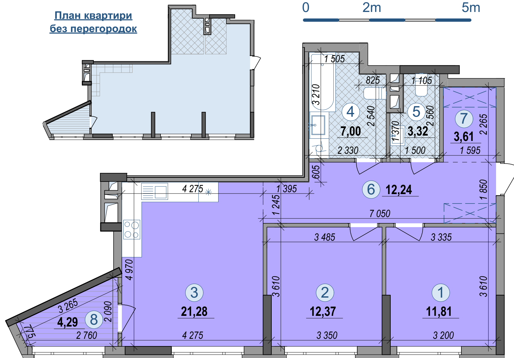
План поверху
