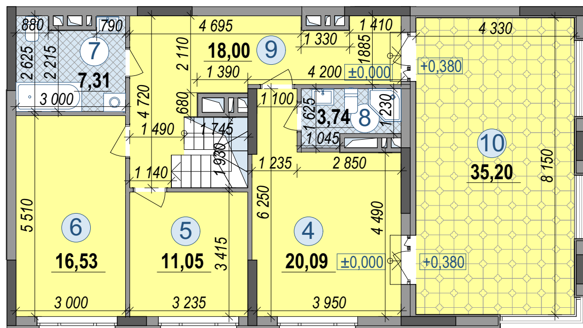
II рівень
