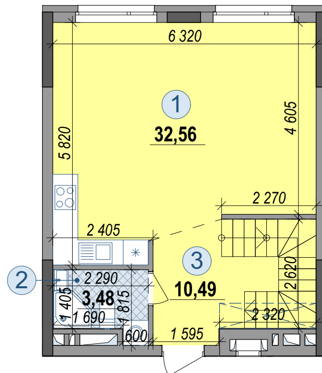
I рівень
