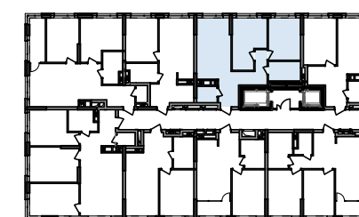
План поверху
