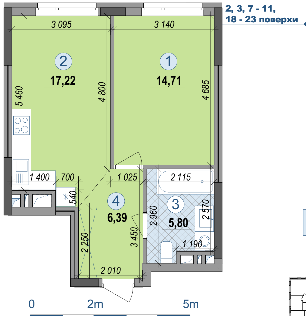
План поверху
